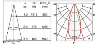
CREE COB 8W-36°
