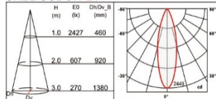
CREE COB 8W-24°
