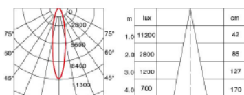
35W 24° 3000K CRI>90
