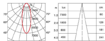
35W 36° 3000K CRI>90
