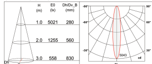
CREE COB 8W-15°
