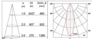
CREE COB 8W-24°
