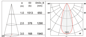
CREE COB 8W-36°
